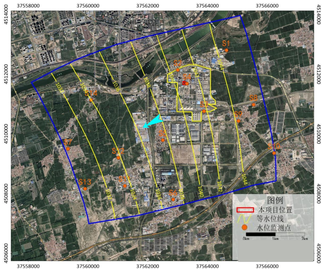
图3.2-1 枯水期区域等水位线图
