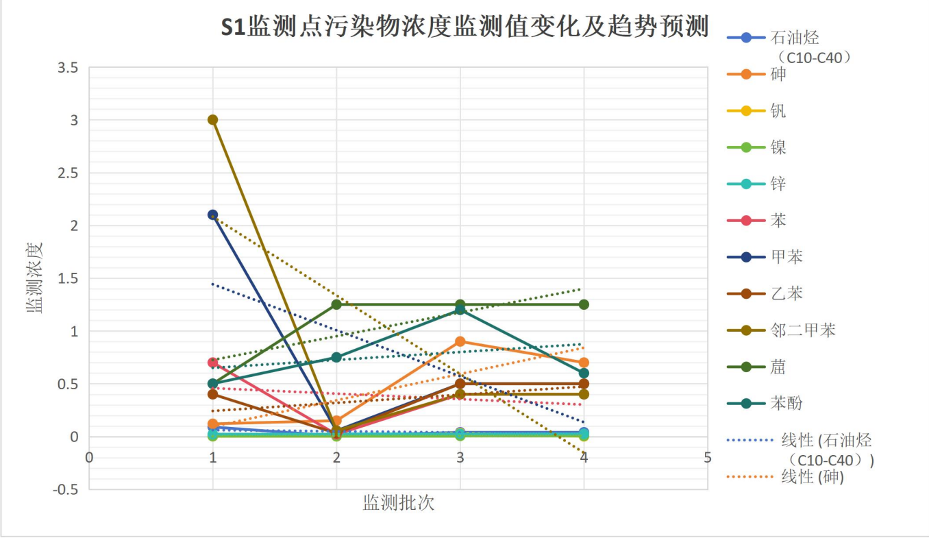
图8.2-2 S1监测点污染物监测值变化及趋势预测图
