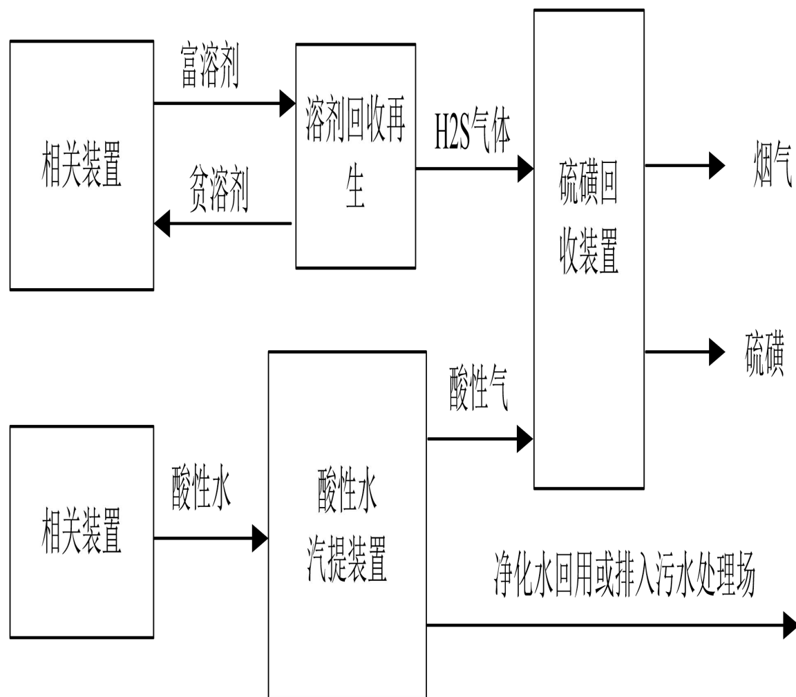
图4.1-1 全厂生产加工流程进出物料情况示意图
