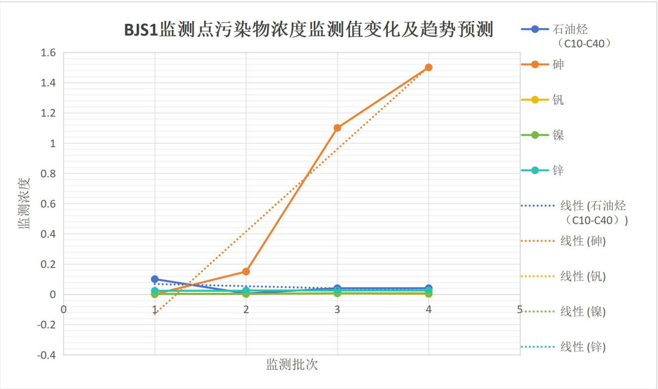
图8.2-1 对照采样点污染物监测值变化及趋势预测图
