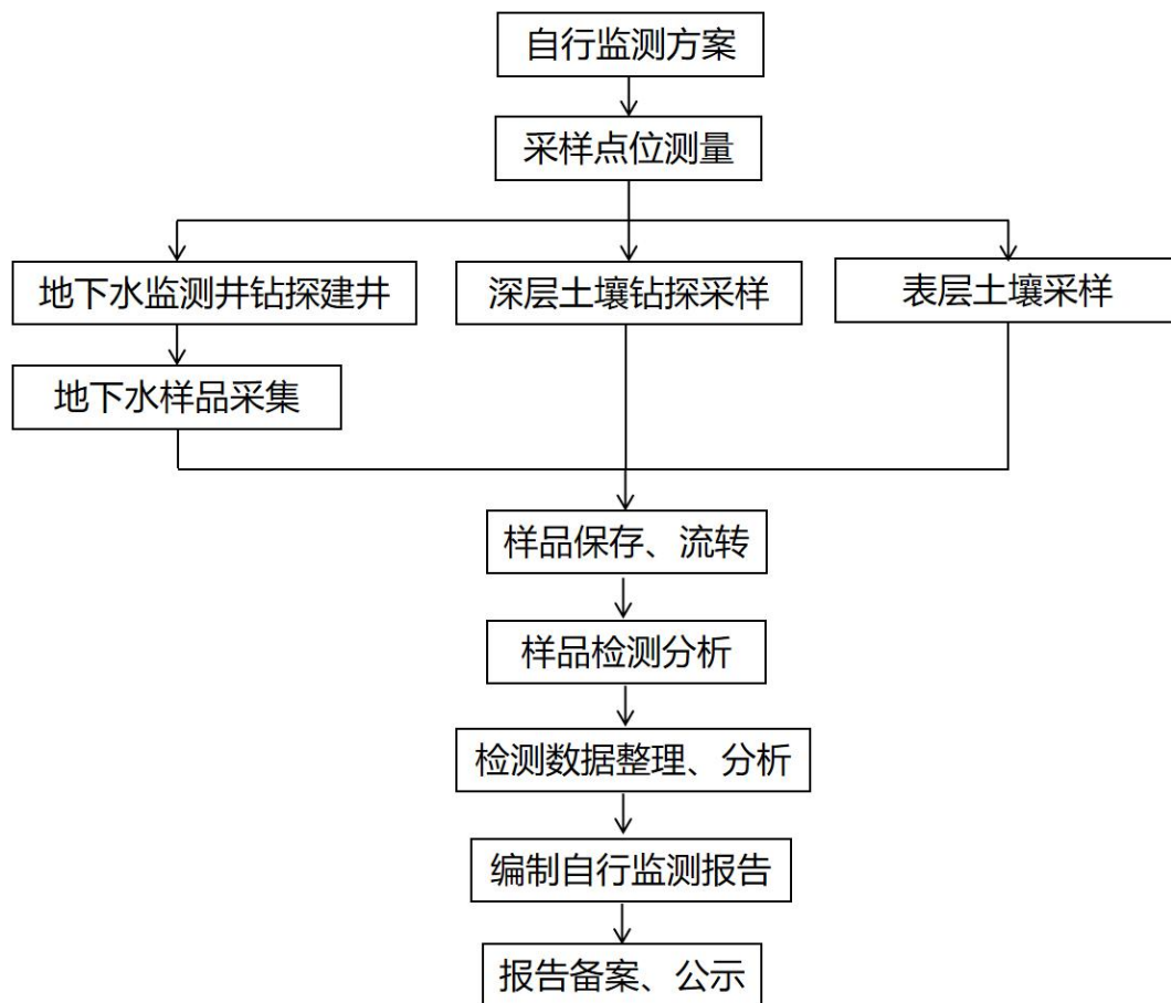
图1.3-3 自行监测工作流程图
