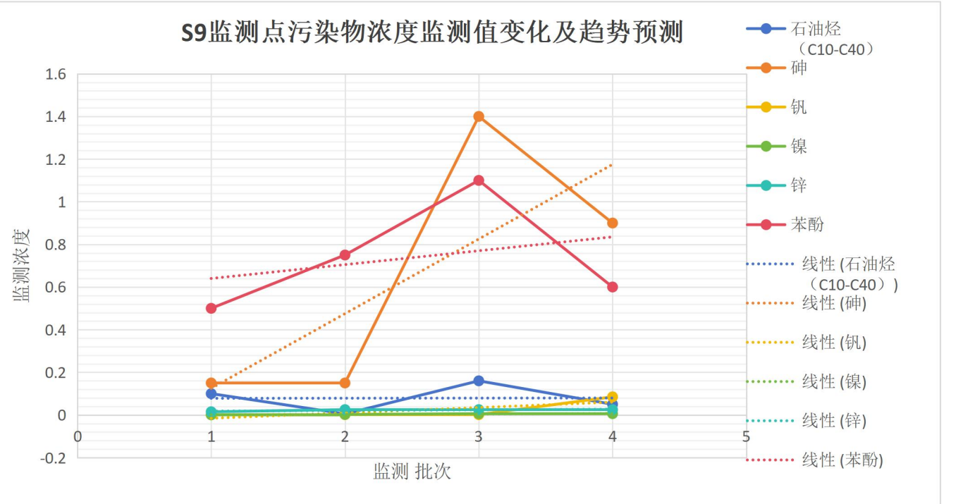
图8.2-4 S9监测点污染物监测值变化及趋势预测图
