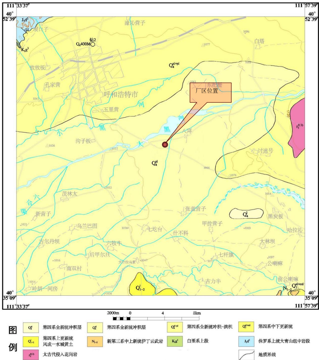
图3. 1-1 区域地质图
